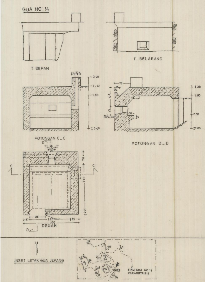
Gambar 4. Denah dan potongan Gua Jepang Nomor 18 (sebelum penomoran ulang tahun 2016 disebut Gua Jepang Nomor 14) (Sumber: Suaka Peninggalan Sejarah dan Purbakala Daerah Istimewa Yogyakarta, 2000)
